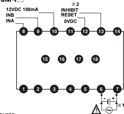
○ CT6M-I □
