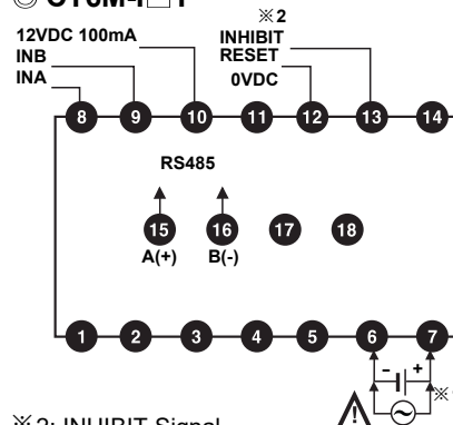
○ CT6M-I □ T
